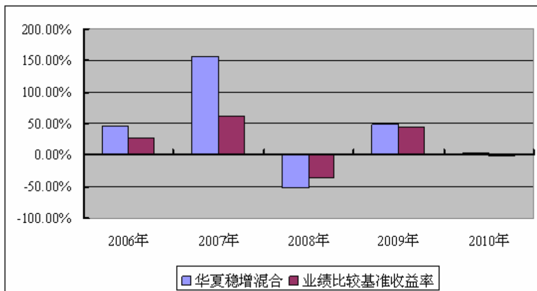
华夏平稳增长混合型证券投资基金 自基金转型以来每年净值增长率图
