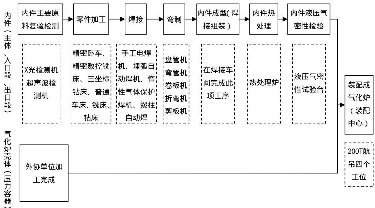
气化炉生产工艺流程
