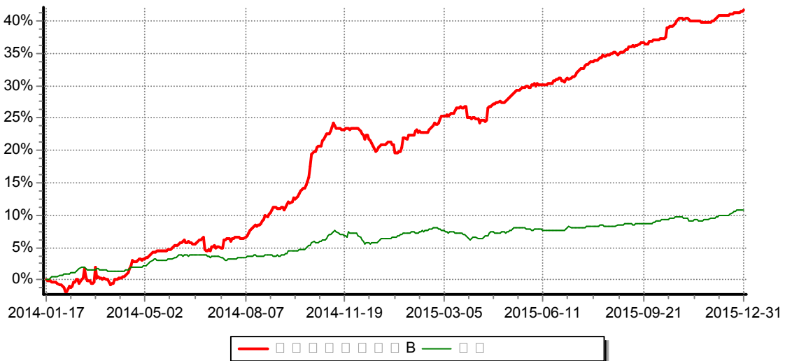
累计净值增长率与业绩比较基准收益率历史走势对比图 (2014年1月17日-2015年12月31日)
