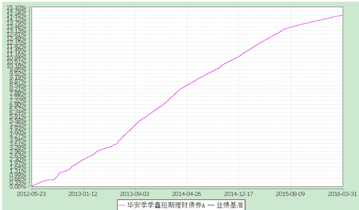
华安季季鑫短期理财债券型证券投资基金 累计净值收益率与业绩比较基准收益率历史走势对比图 (2012 年 5 月 23 日至 2016 年 3 月 31 日)
