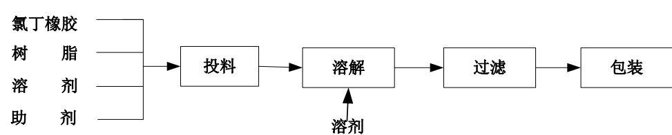
3、胶粘剂生产流程图
