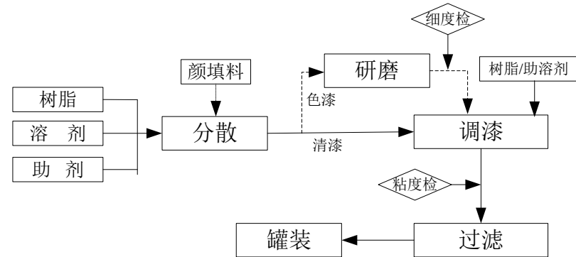
硝基漆、聚氨酯漆生产工艺流程
