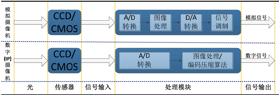
模拟摄像机与数字摄像机的比较
