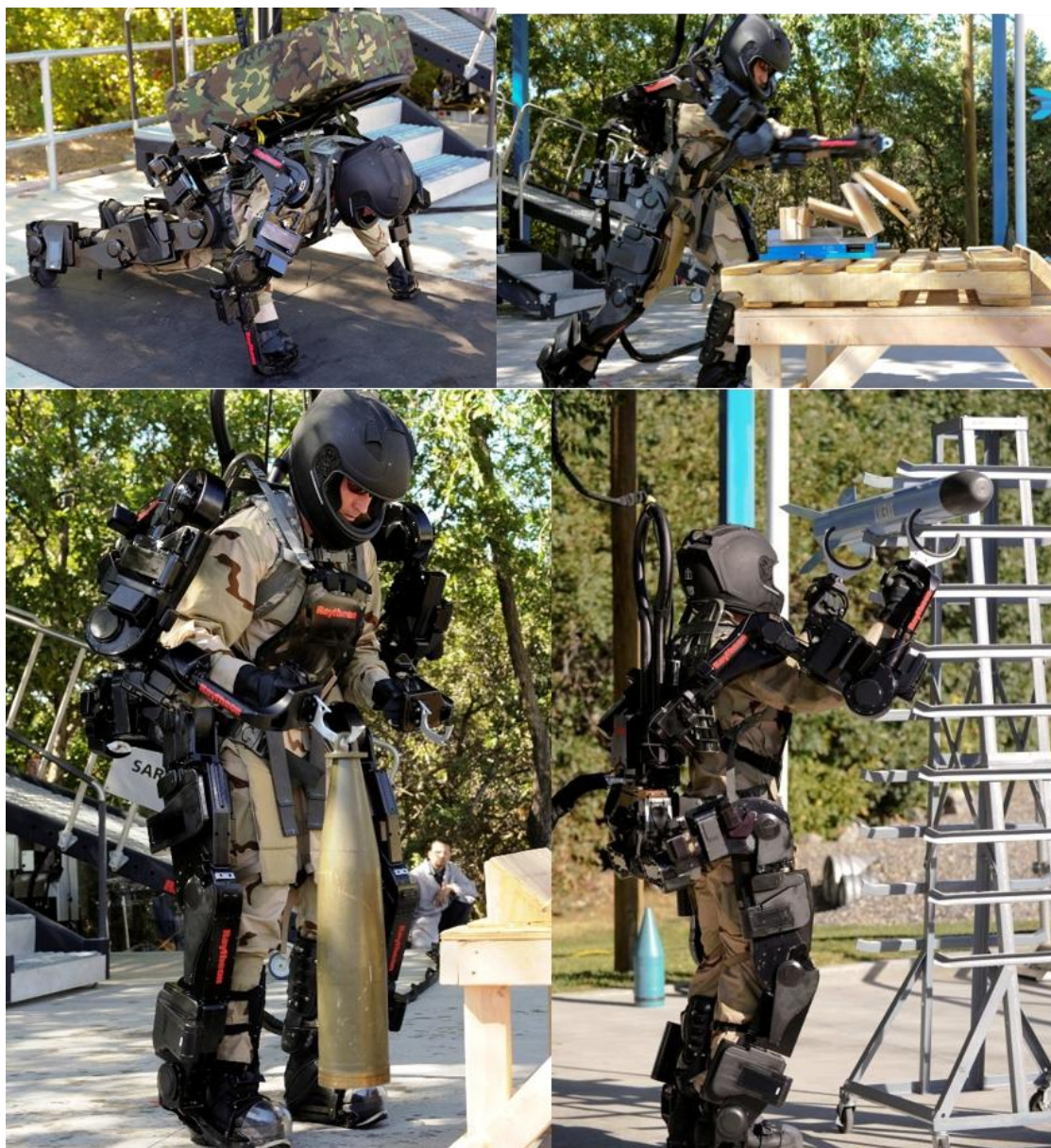
图 3: 美国 Raytheon Sarcos XOS 2 外骨骼机器人进行负重、击打演示，可进行 100 升背包负重、单手提起 155 毫米榴弹炮弹药等
