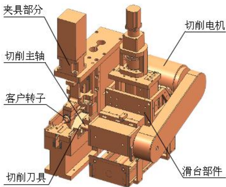
切削装置
