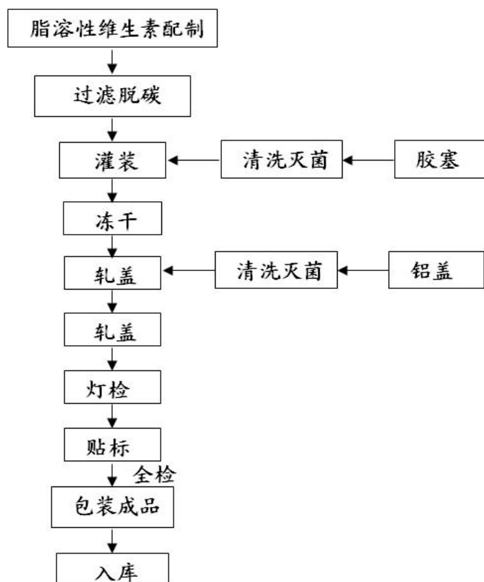
3) 注射用多种维生素冻干粉针生产工艺流程图
