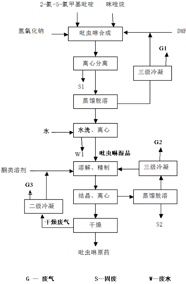
2. 吡虫啉原药生产流程图
