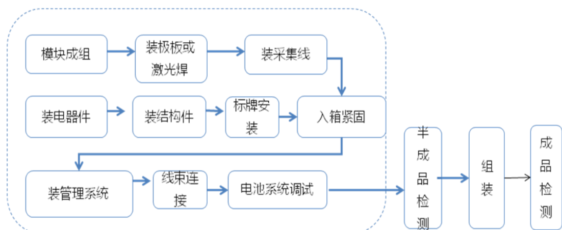
● PACK 生产工艺流程图
