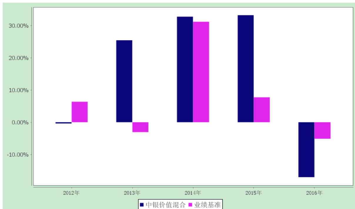
中银价值精选灵活配置混合型证券投资基金 过去五年基金净值增长率与业绩比较基准收益率的对比图
