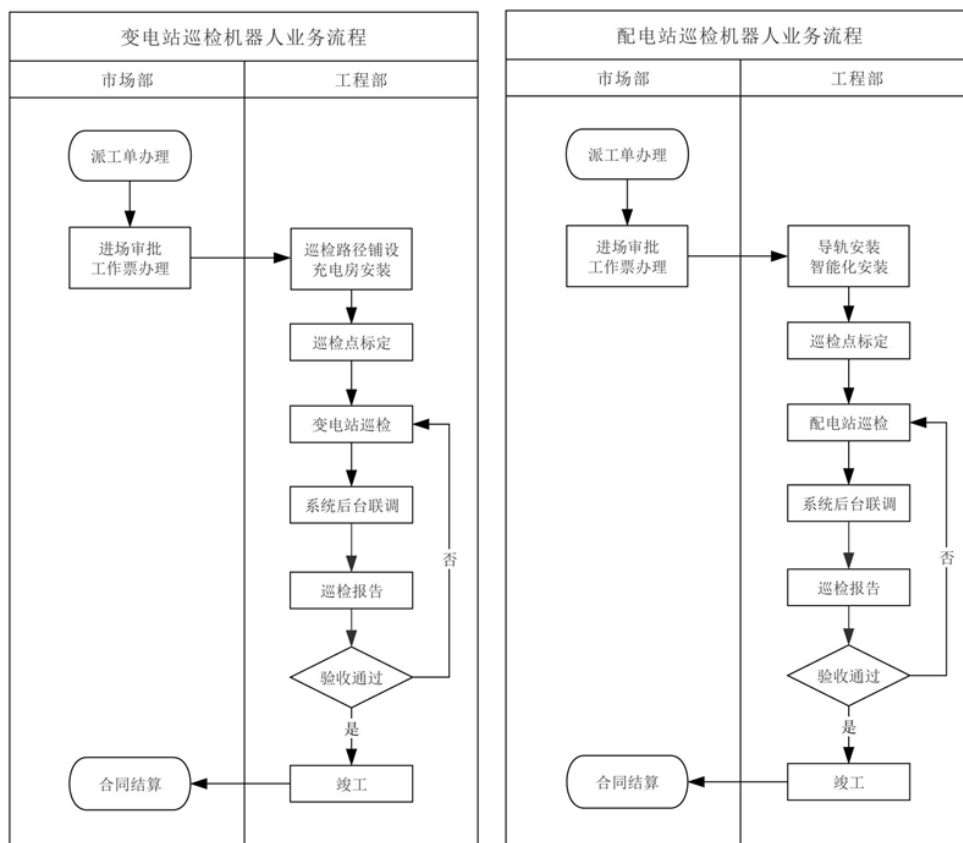
智能巡检机器人施工流程图
