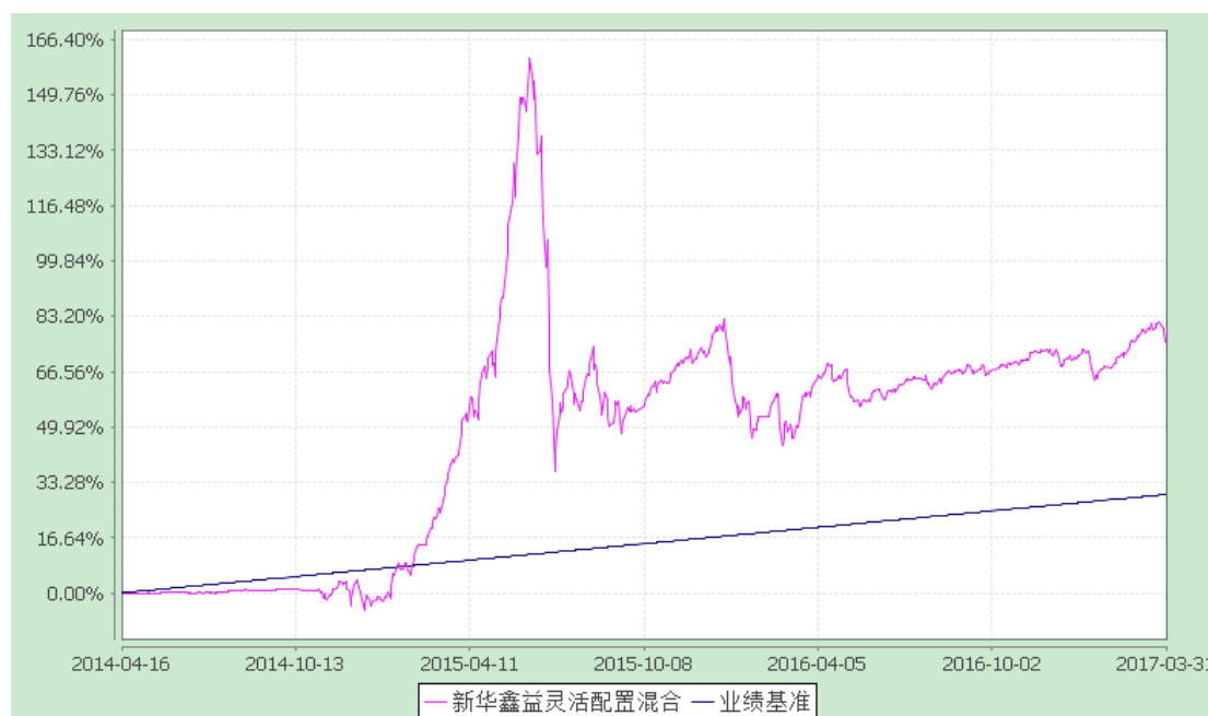
新华鑫益灵活配置混合型证券投资基金 累计净值增长率与业绩比较基准收益率历史走势对比图 (2014 年 4 月 16 日至 2017 年 3 月 31 日)
