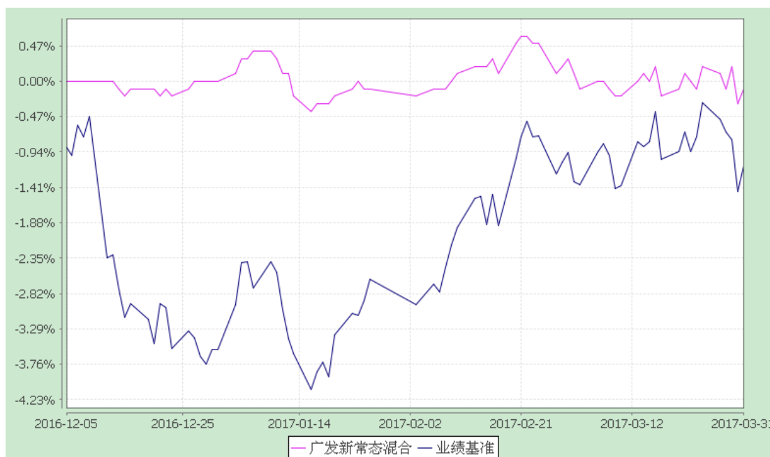
广发新常态灵活配置混合型证券投资基金 累计净值增长率与业绩比较基准收益率历史走势对比图 (2016 年 12 月 5 日至 2017 年 3 月 31 日)
