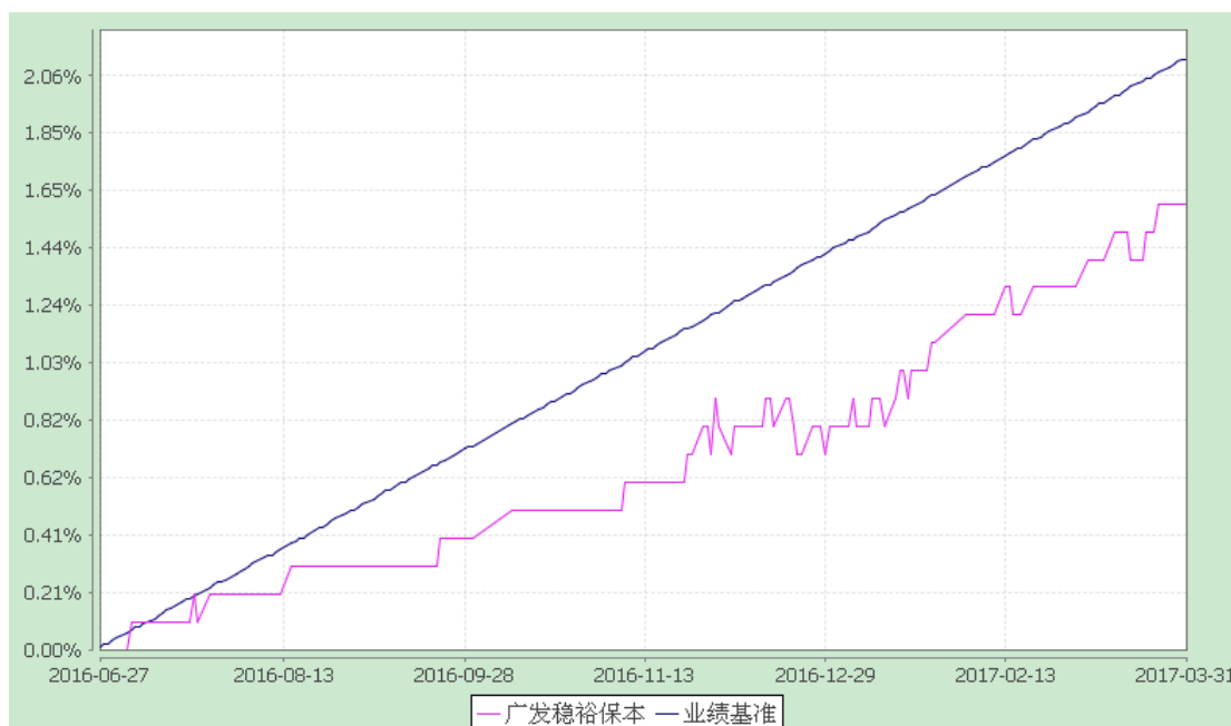
广发稳裕保本混合型证券投资基金 累计净值增长率与业绩比较基准收益率历史走势对比图 (2016 年 6 月 27 日至 2017 年 3 月 31 日)
