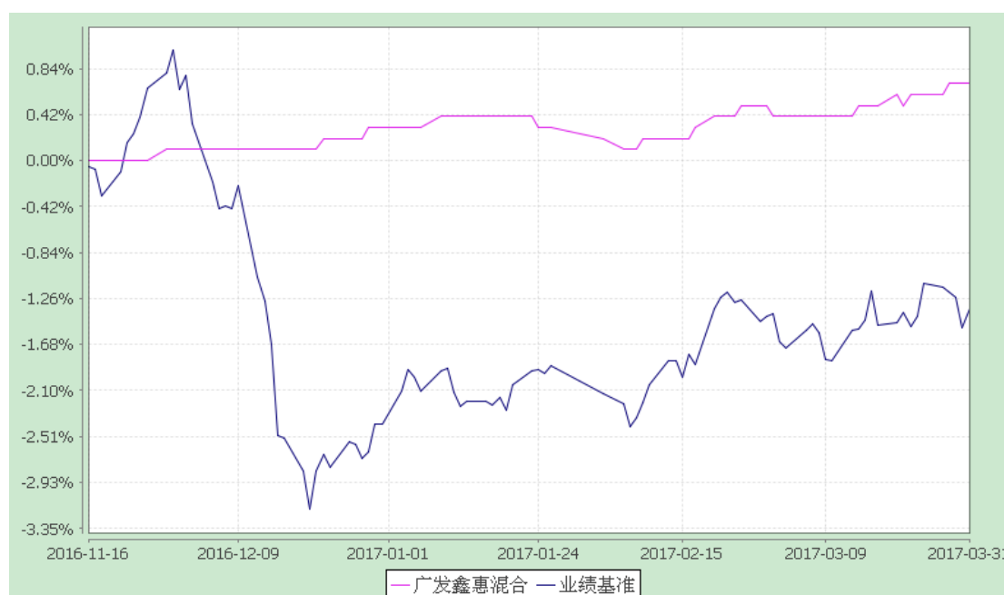
广发鑫惠灵活配置混合型证券投资基金 累计净值增长率与业绩比较基准收益率历史走势对比图 (2016 年 11 月 16 日至 2017 年 3 月 31 日)
