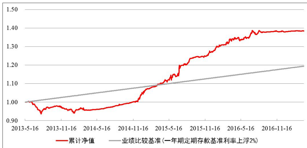
集合计划累计份额净值增长率与业绩基准收益率的历史走势对比图 (2013年5月16日至2017年3月31日)
