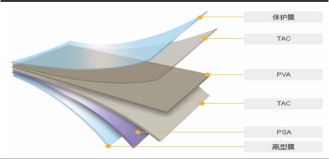
偏光片的基本结构
