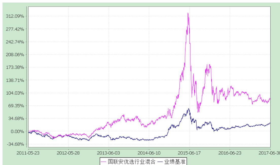
国联安优选行业混合型证券投资基金 累计净值增长率与业绩比较基准收益率历史走势对比图 (2011年5月23日至2017年6月30日)
