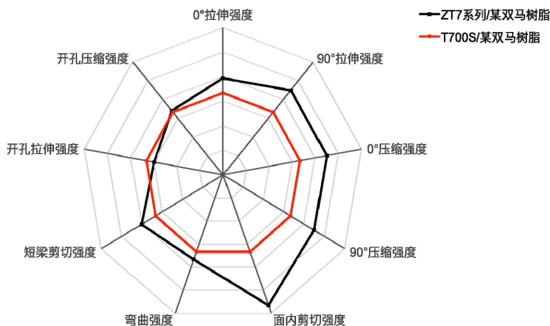
图6-26: ZT7系列牌号与日本东丽T700S级碳纤维生产的复合材料相关性性能指标对比图
