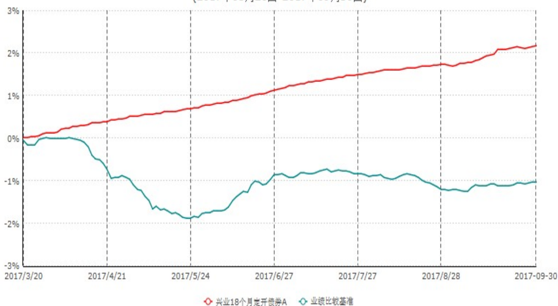
兴业18个月定开债券A累计净值增长率与业绩比较基准收益率历史走势对比图 (2017年03月20日-2017年09月30日)
