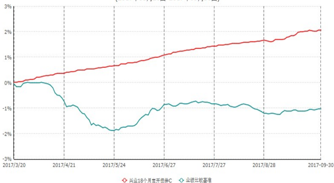
兴业18个月定开债券C累计净值增长率与业绩比较基准收益率历史走势对比图 (2017年03月20日-2017年09月30日)
