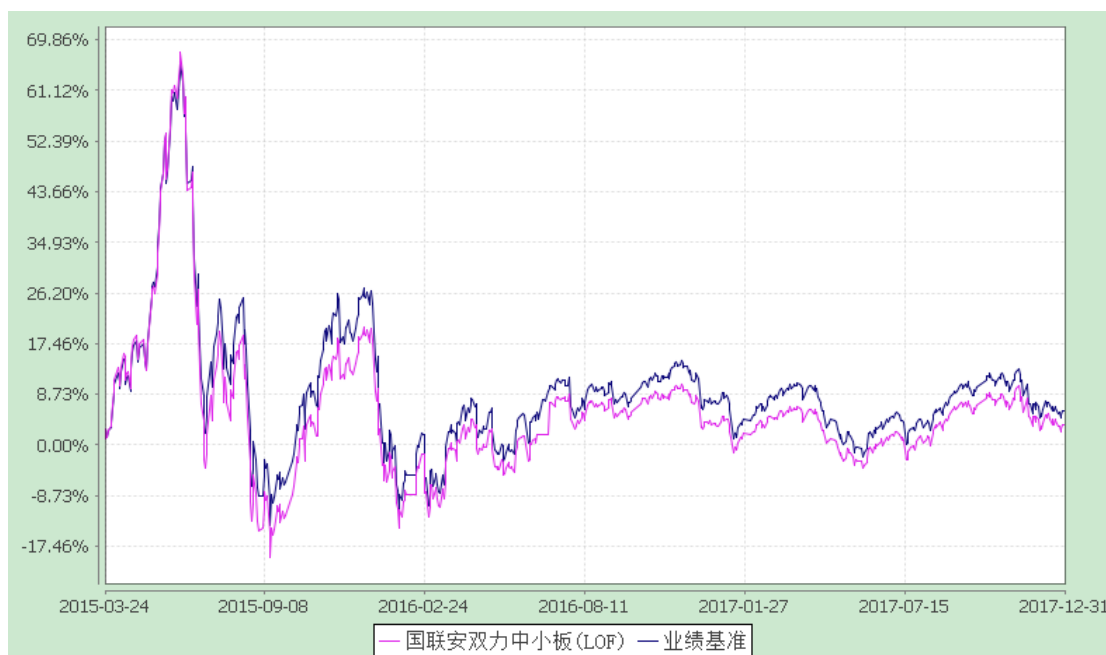
国联安双力中小板综指证券投资基金(LOF) 累计净值增长率与业绩比较基准收益率历史走势对比图 (2015年3月24日至2017年12月31日)
