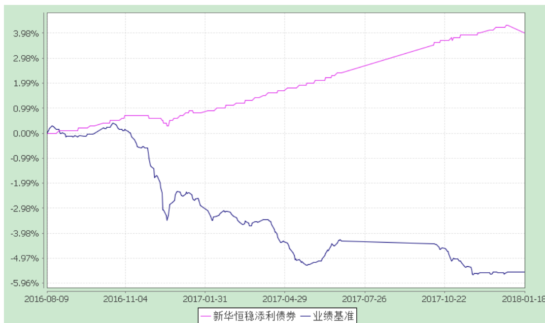
新华恒稳添利债券型证券投资基金 累计净值增长率与业绩比较基准收益率历史走势对比图 (2016 年 8 月 9 日至 2017 年 12 月 31 日)
