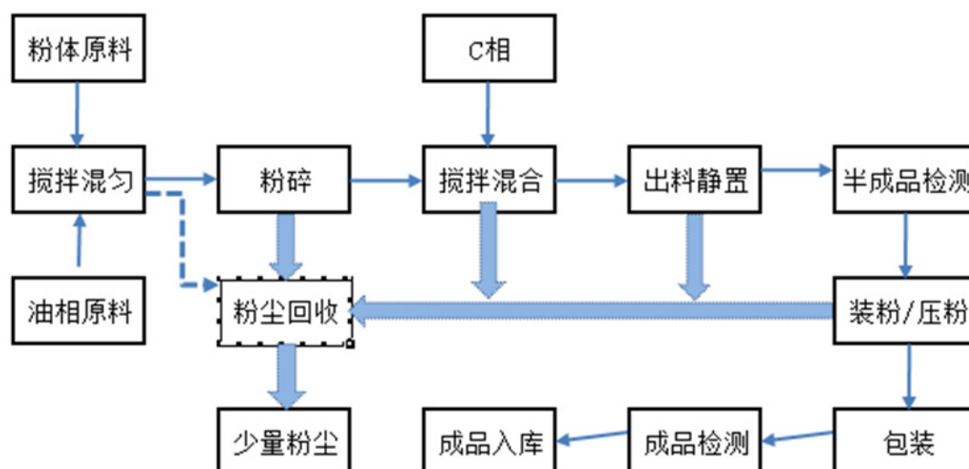
(2) 化妆粉饼生产工艺流程图
