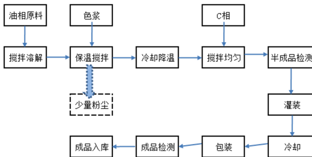
(1) 蜡基产品生产工艺流程图
