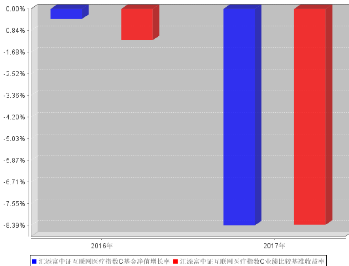
汇添富中证互联网医疗指数C自基金合同生效以来基金每年净值增长率及其与同期业绩比较基准收益率的对比图
