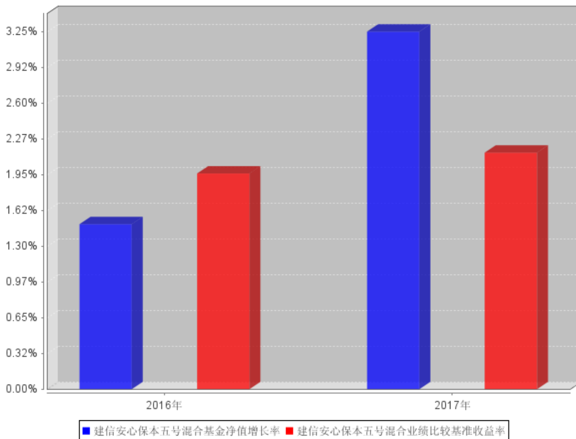
建信安心保本五号混合自基金合同生效以来基金每年净值增长率及其与同期业绩比较基准收益率的对比图
