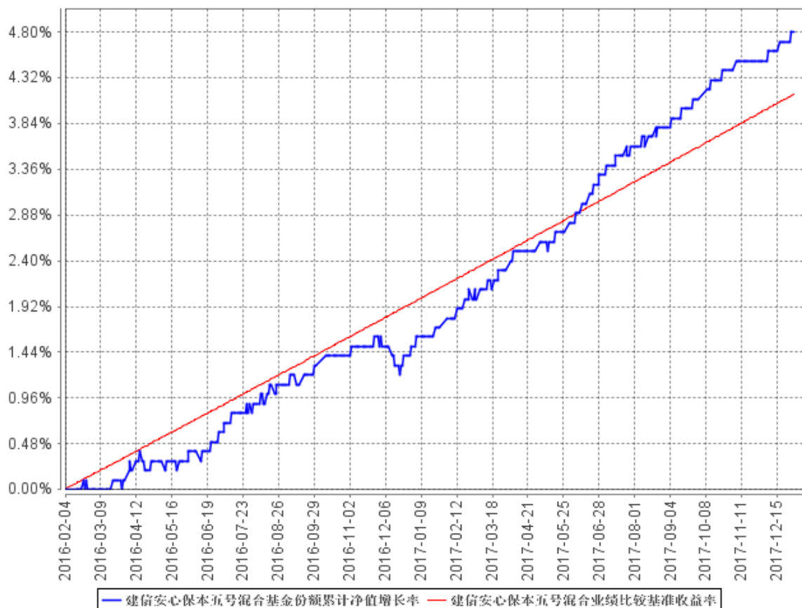
建信安心保本五号混合基金份额累计净值增长率与同期业绩比较基准收益率的历史走势对比图
