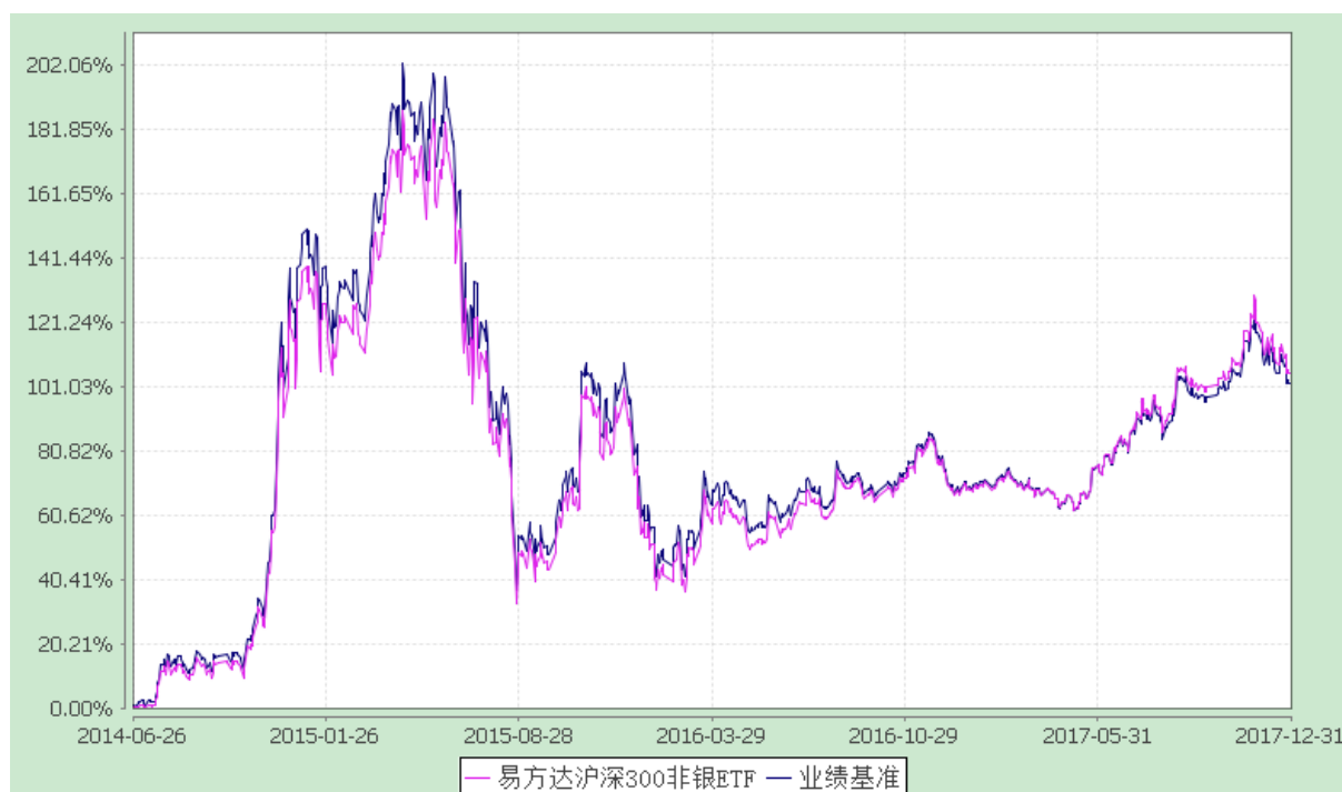
易方达沪深 300 非银行金融交易型开放式指数证券投资基金 份额累计净值增长率与业绩比较基准收益率历史走势对比图 (2014 年 6 月 26 日至 2017 年 12 月 31 日)
