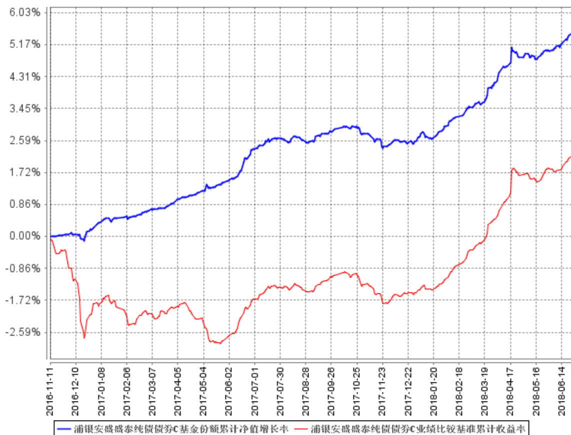
浦银安盛盛泰纯债债券C基金份额累计净值增长率与同期业绩比较基准收益率的历史走势对比图
