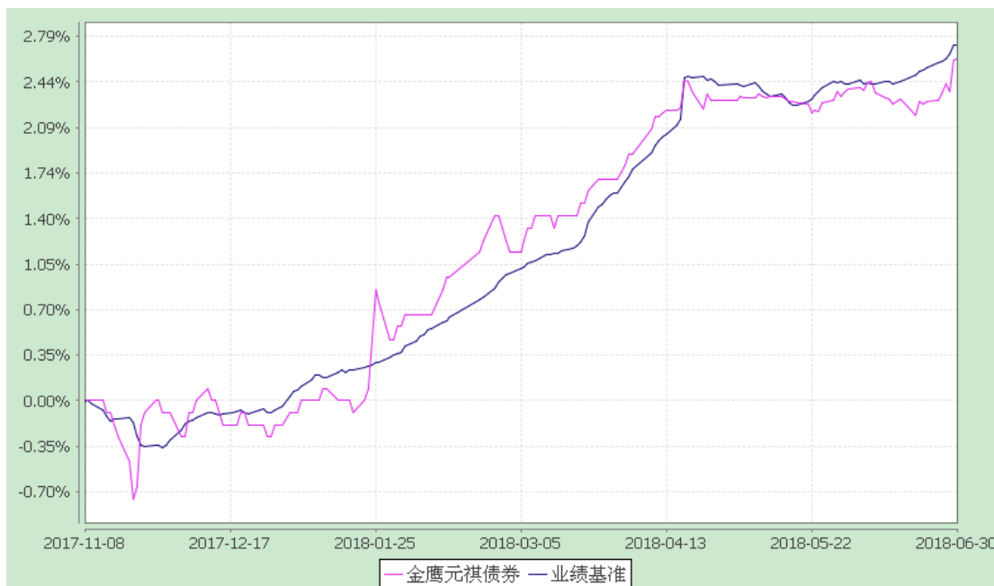
金鹰元祺信用债债券型证券投资基金 累计净值增长率与业绩比较基准收益率历史走势对比图 (2017 年 11 月 8 日至 2018 年 6 月 30 日)
