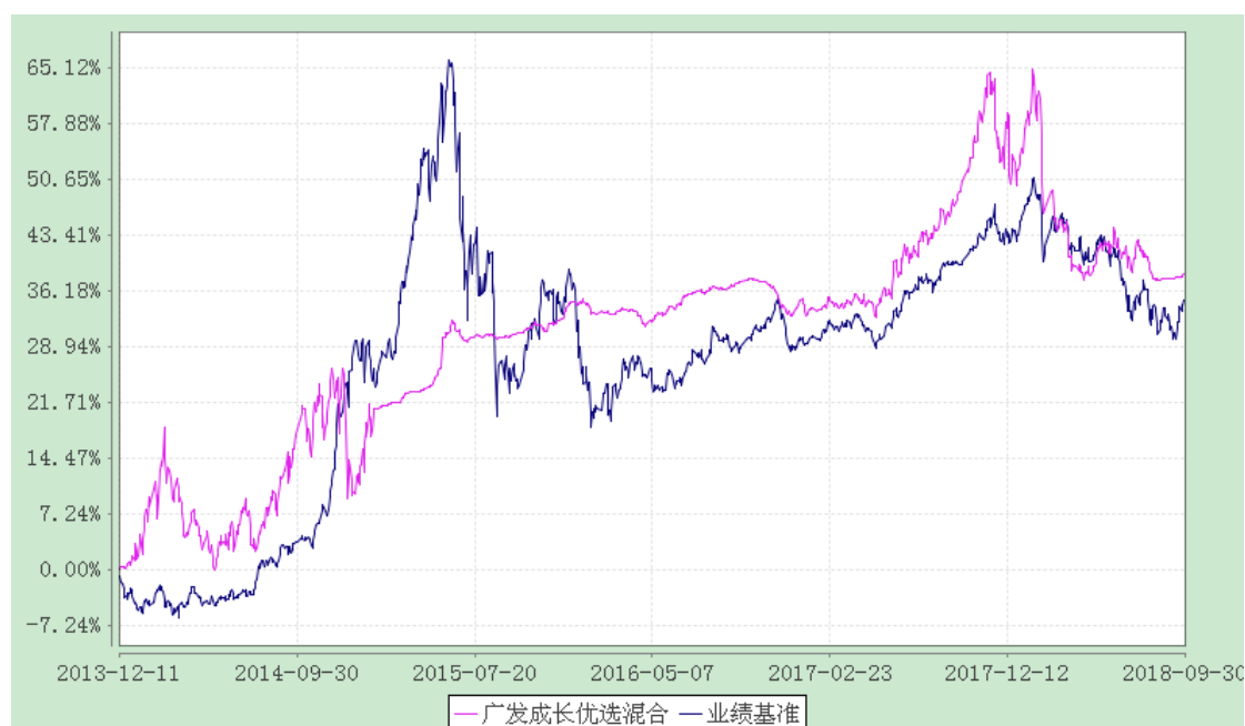
广发成长优选灵活配置混合型证券投资基金 累计净值增长率与业绩比较基准收益率历史走势对比图 (2013 年 12 月 11 日至 2018 年 9 月 30 日)
