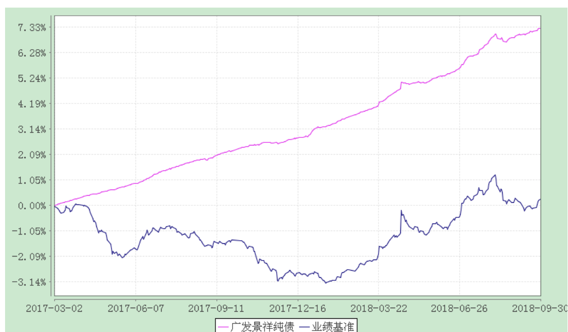
广发景祥纯债债券型证券投资基金 累计净值增长率与业绩比较基准收益率历史走势对比图 (2017 年 3 月 2 日至 2018 年 9 月 30 日)
