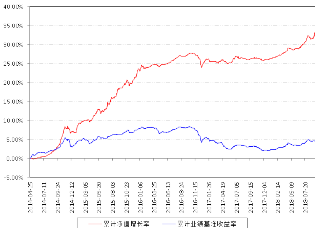
南方通利债券A累计净值增长率与同期业绩比较基准收益率的历史走势 对比图
