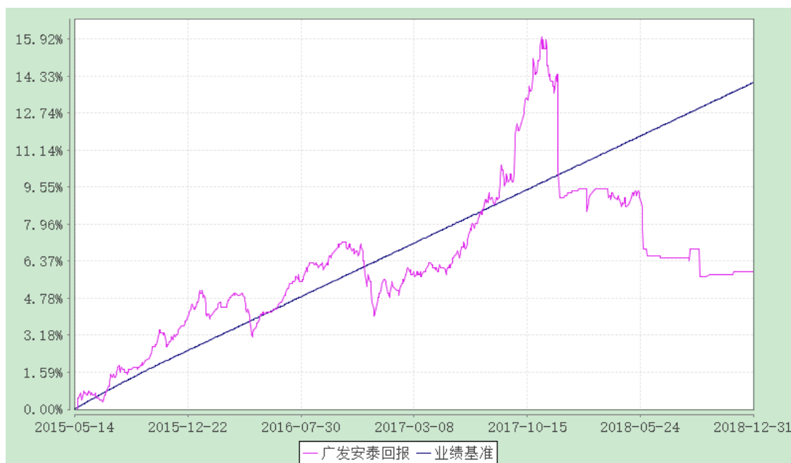
广发安泰回报混合型证券投资基金 累计净值增长率与业绩比较基准收益率历史走势对比图 (2015 年 5 月 14 日至 2018 年 12 月 31 日)
