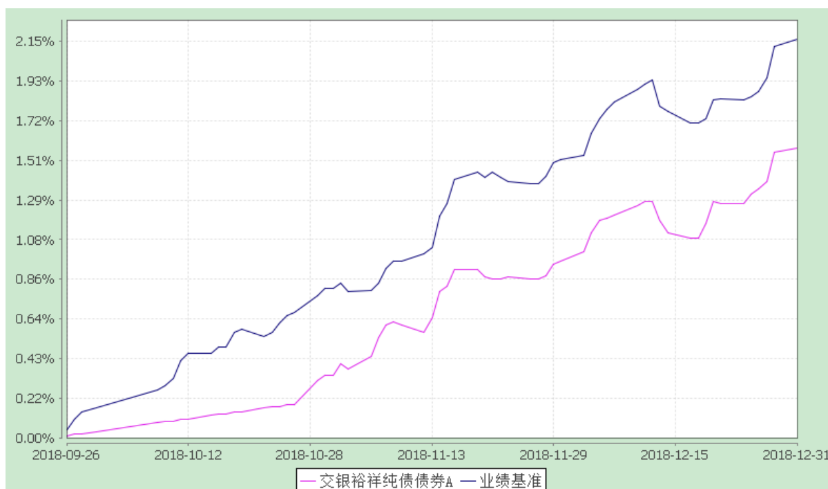
交银施罗德裕祥纯债债券型证券投资基金 份额累计净值增长率与业绩比较基准收益率的历史走势对比图 (2018年9月26日至2018年12月31日)
