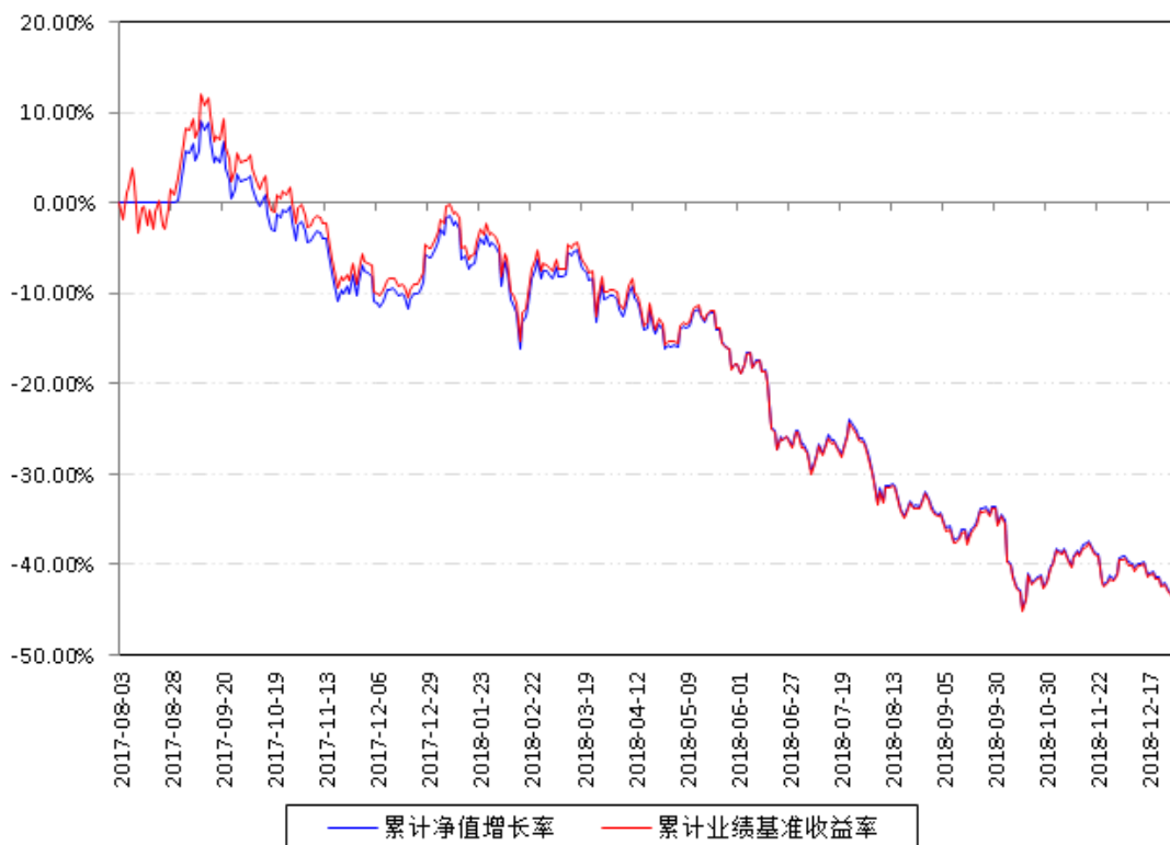
南方中证申万有色金属ETF累计净值增长率与同期业绩比较基准收益率的历史走势对比图
