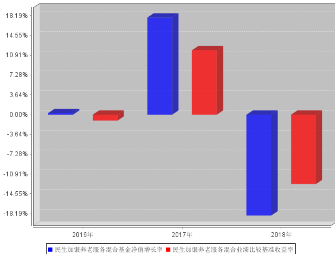
民生加银养老服务混合自基金合同生效以来基金每年净值增长率及其与同期业绩比较基准收益率的对比图
