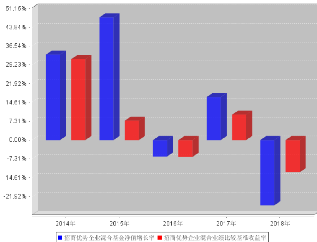
招商优势企业混合过去五年基金每年净值增长率及其与同期业绩比较基准收益率的对比图
