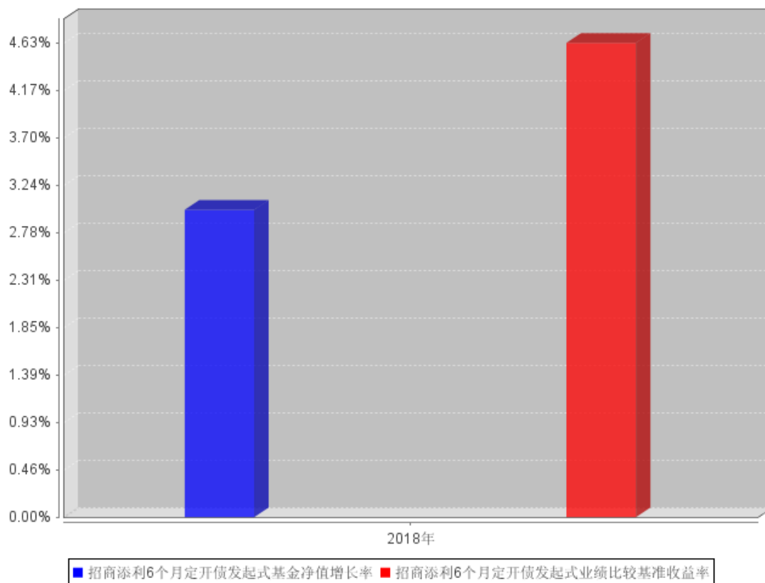
招商添利6个月定开债发起式自基金合同生效以来基金每年净值增长率及其与同期业绩比较基准收益率的对比图
