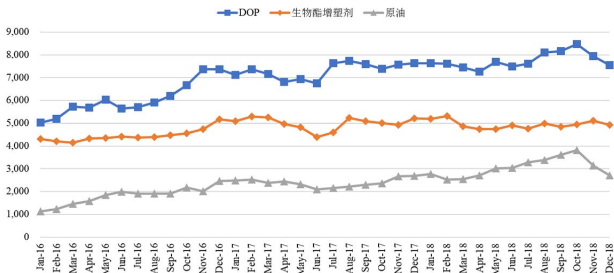
2016-2018年公司生物酯增塑剂售价与DOP价格、原油价格走势对比（元/吨）
