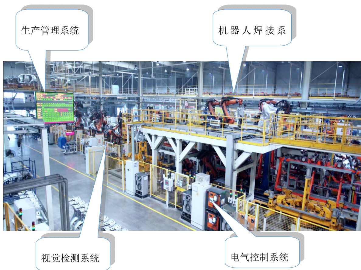
（1）焊装自动化生产线整线实物图
