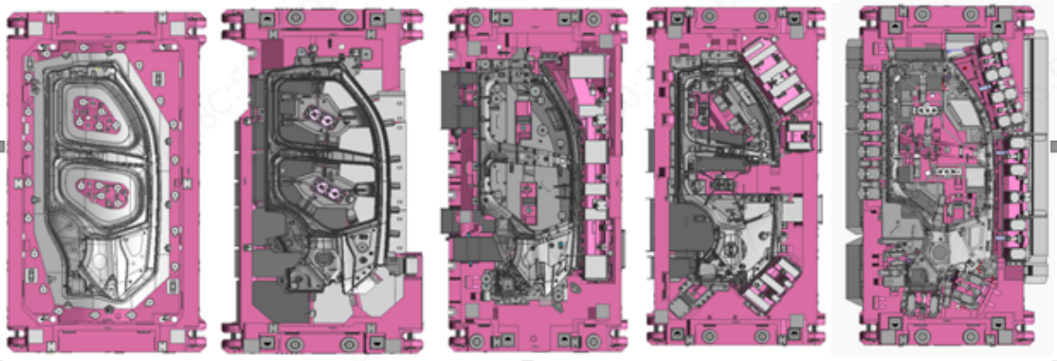
冲压工序一模具 冲压工序二模具 冲压工序三模具 冲压工序四模具 冲压工序五模具
