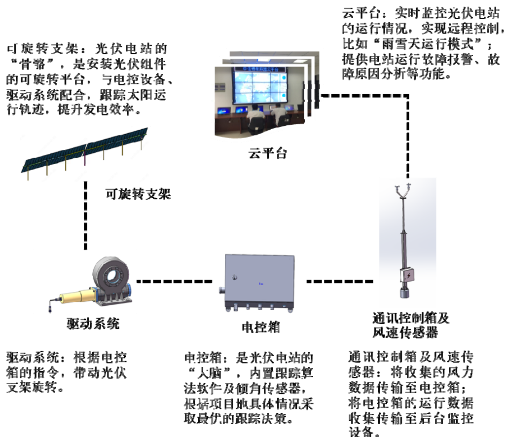
跟踪支架产品示意图
