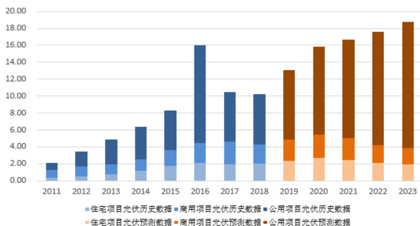
美国并网项目按类型划分 (单位: 吉瓦)
