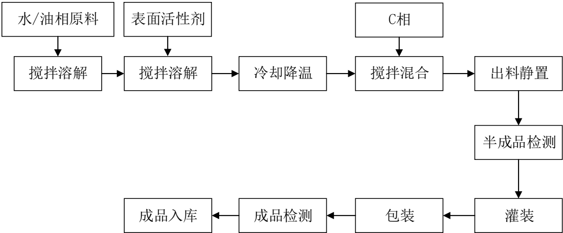
（5）一般液态单元-卸妆产品生产工艺流程图
