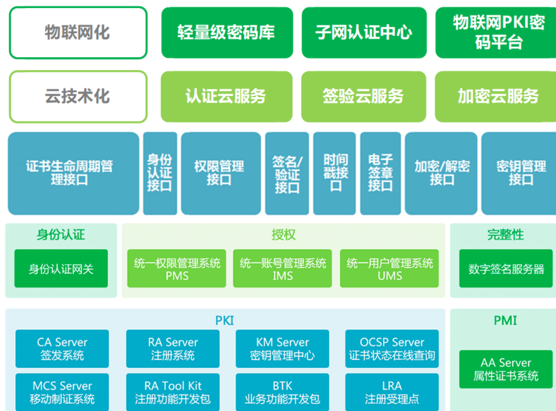
新一代应用安全支撑平台产品结构图
