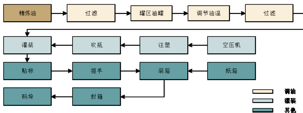
(3) 小包装食用油工艺流程图
