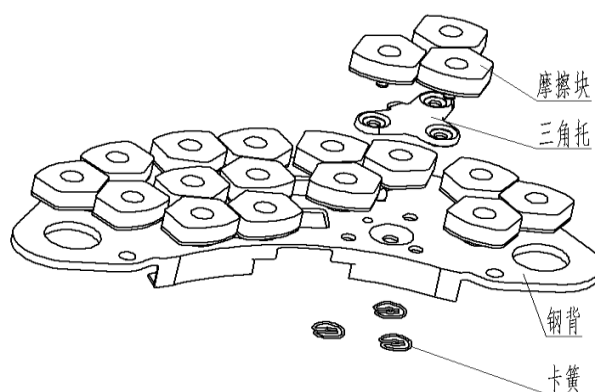
粉末冶金闸片结构与外形示意图
