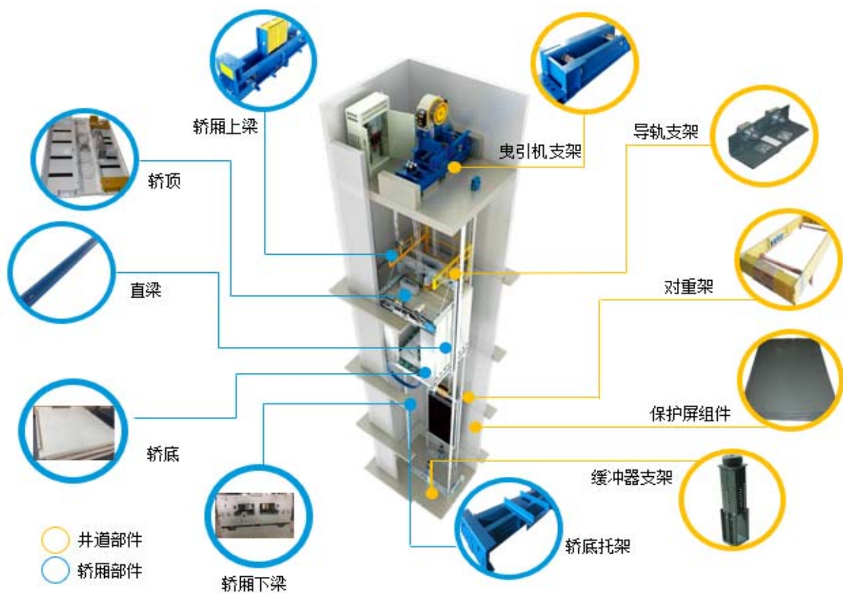
发行人直梯主要产品示意图
