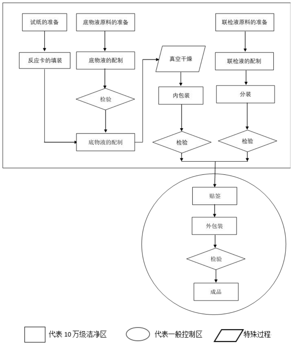
图 6-11 干化学诊断试剂工艺流程
