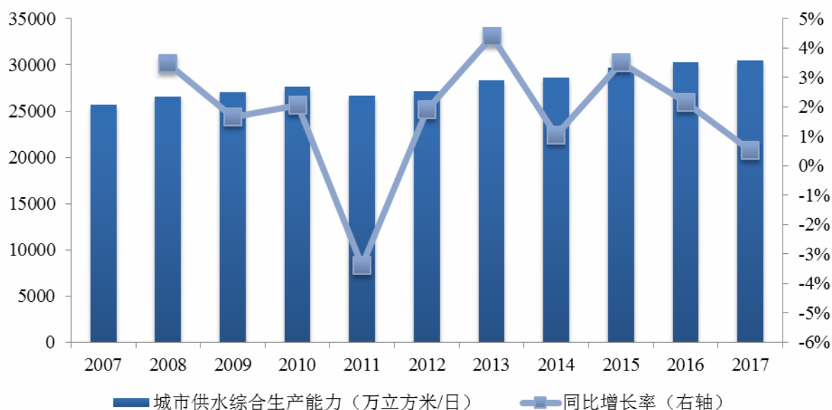
2007年至2017年全国城市供水综合生产能力情况
