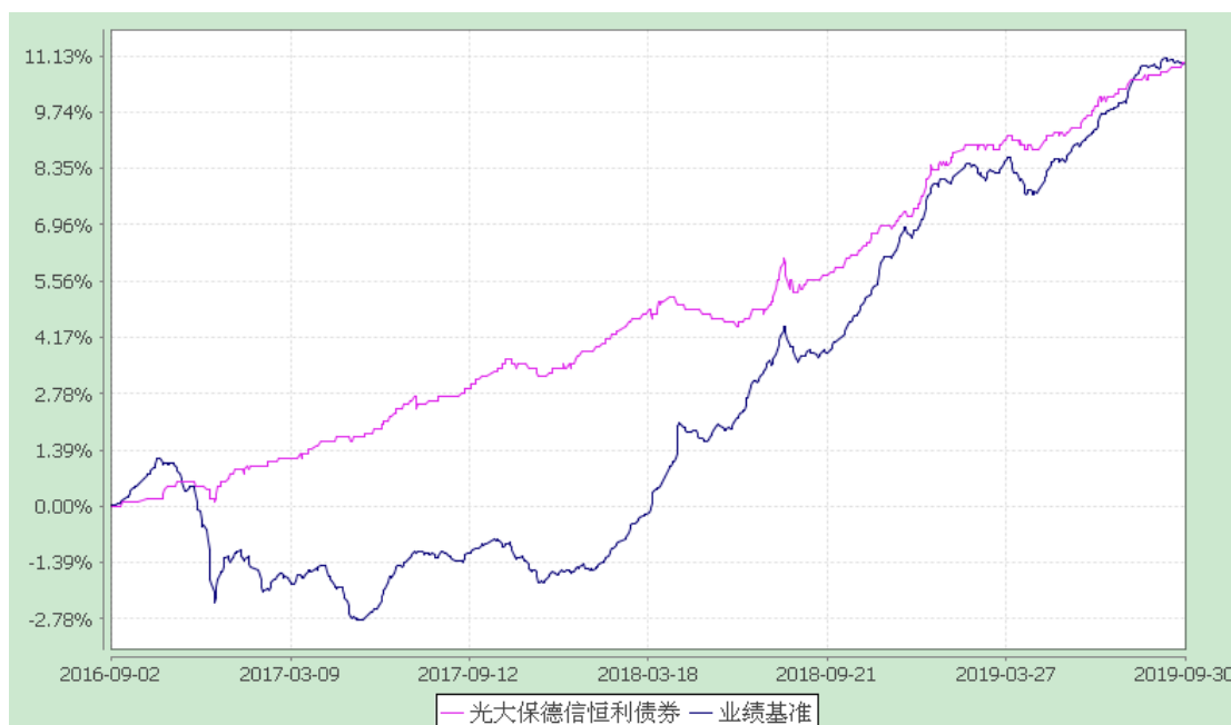
光大保德信恒利纯债债券型证券投资基金 累计净值增长率与业绩比较基准收益率历史走势对比图 (2016年9月2日至2019年9月30日)
